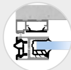
Thin jamb 15 x 35 mm
