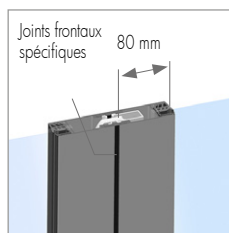
Montant G38 élargi avec intégration de la serrure
