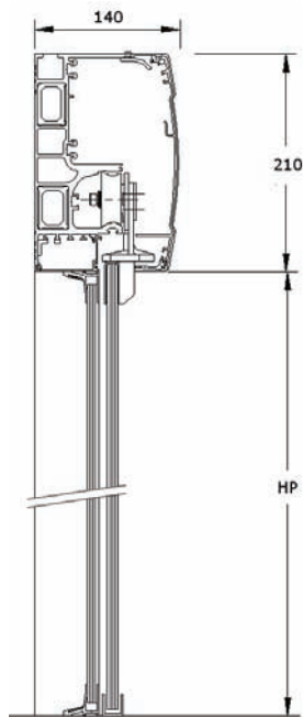
LUMINA avec Fixe Caisson DIVA LC Renforcé
