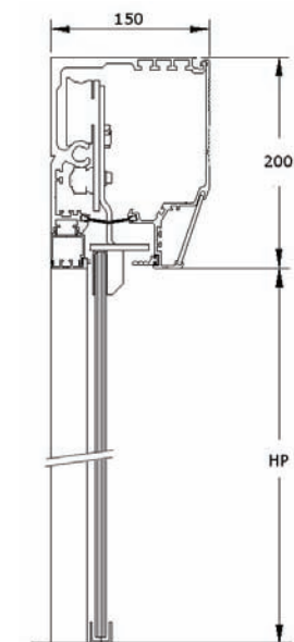
LUMINA Sans Fixe - Caisson DIVA Standard
