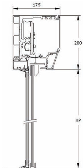
LUMINA Avec Fixe - Caisson DIVA Renforcé
